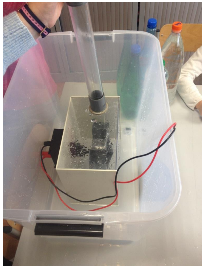
L'énergie hydraulique dans un barrage, modélisée avec un tuyau, un bouchon, une bouteille d'eau.
